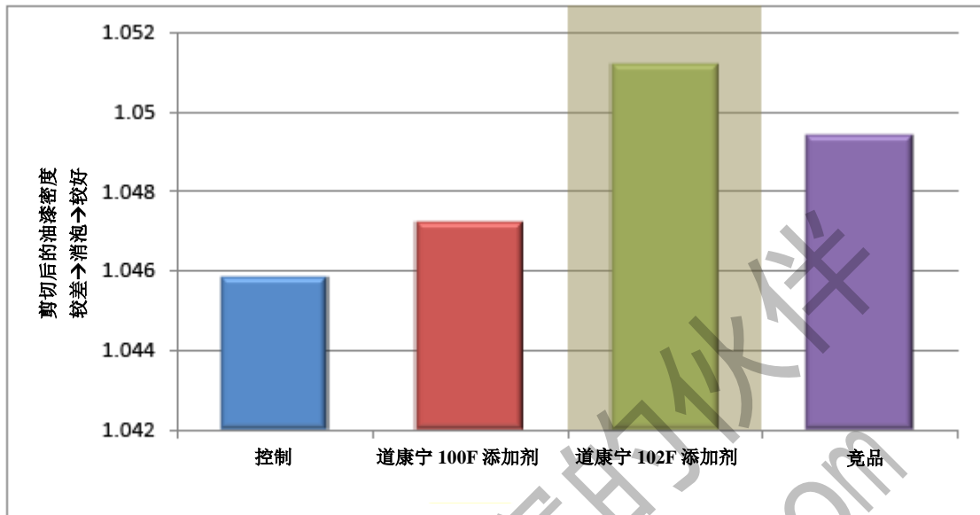
图2: 含交联剂和稀释剂的环氧防护底漆中添加 0.4%含量的道康宁 102F 添加剂。在 1500 转/分的速度下，高速搅拌机剪切 15 分钟后，将等量的油漆倒入扁平的容器中，等待油漆固化。固化后的表面性状显示道康宁 102F 添加剂的消泡性能要强于竞品，采用道康宁 102F 添加剂的表面气泡更少。
